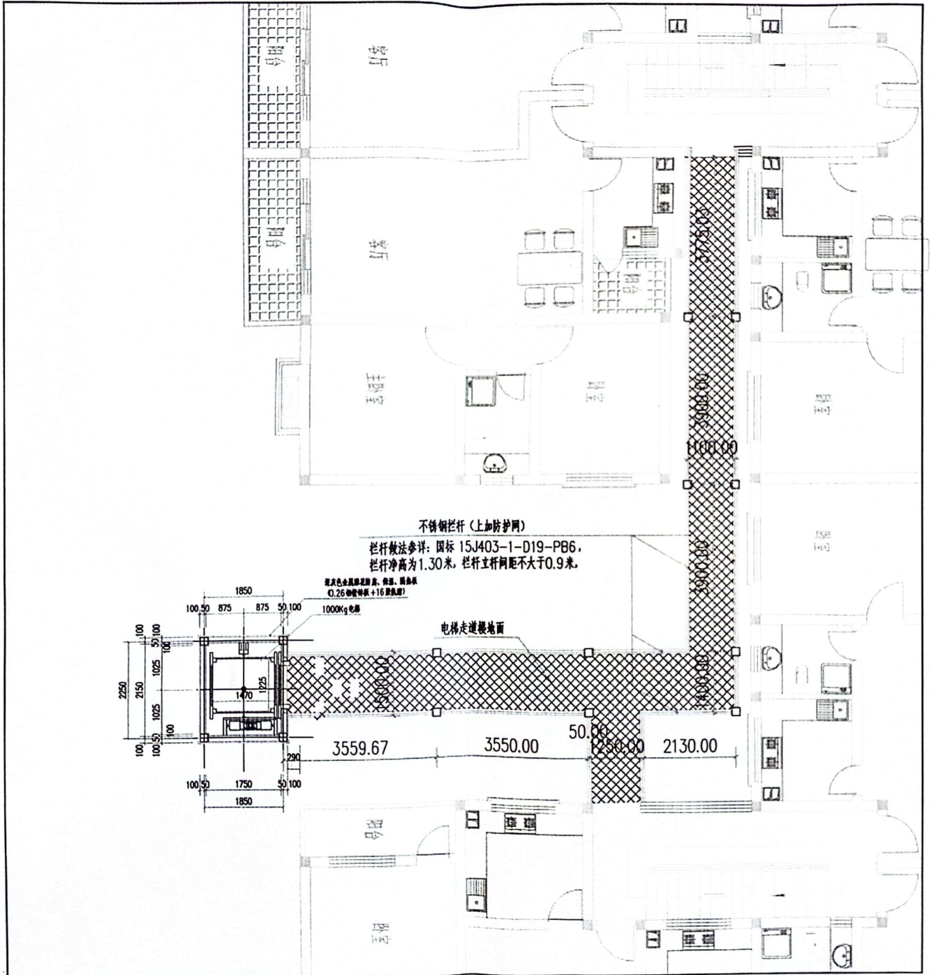
标准层平面图 1:50
